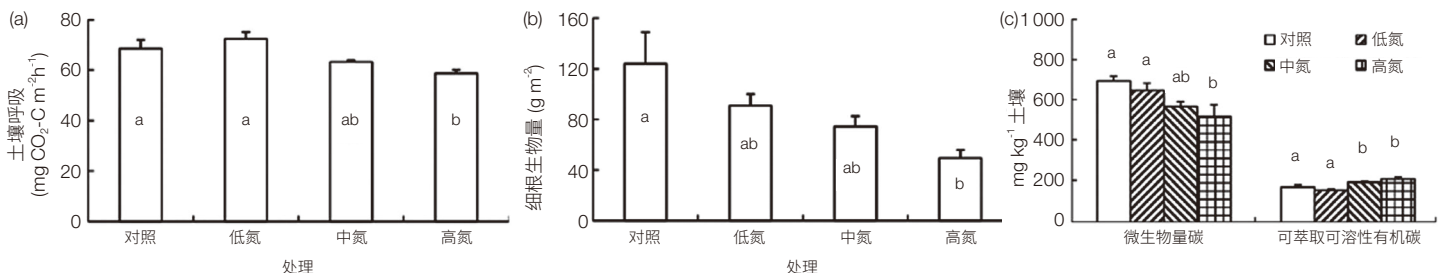
图 3 不同氮添加处理条件下季风常绿阔叶林土壤呼吸 (a)、细根生物量 (b) 和微生物活性 (c) 高氮、中氮和低氮处理喷施氮量分别为 150 \text{ kg ha}^{-1} \text{ yr}^{-1} 、 100 \text{ kg ha}^{-1} \text{ yr}^{-1} 和 50 \text{ kg ha}^{-1} \text{ yr}^{-1}
