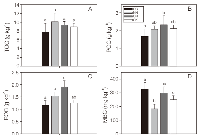
图5 碳-氮交互作用下的土壤各组分有机碳含量
